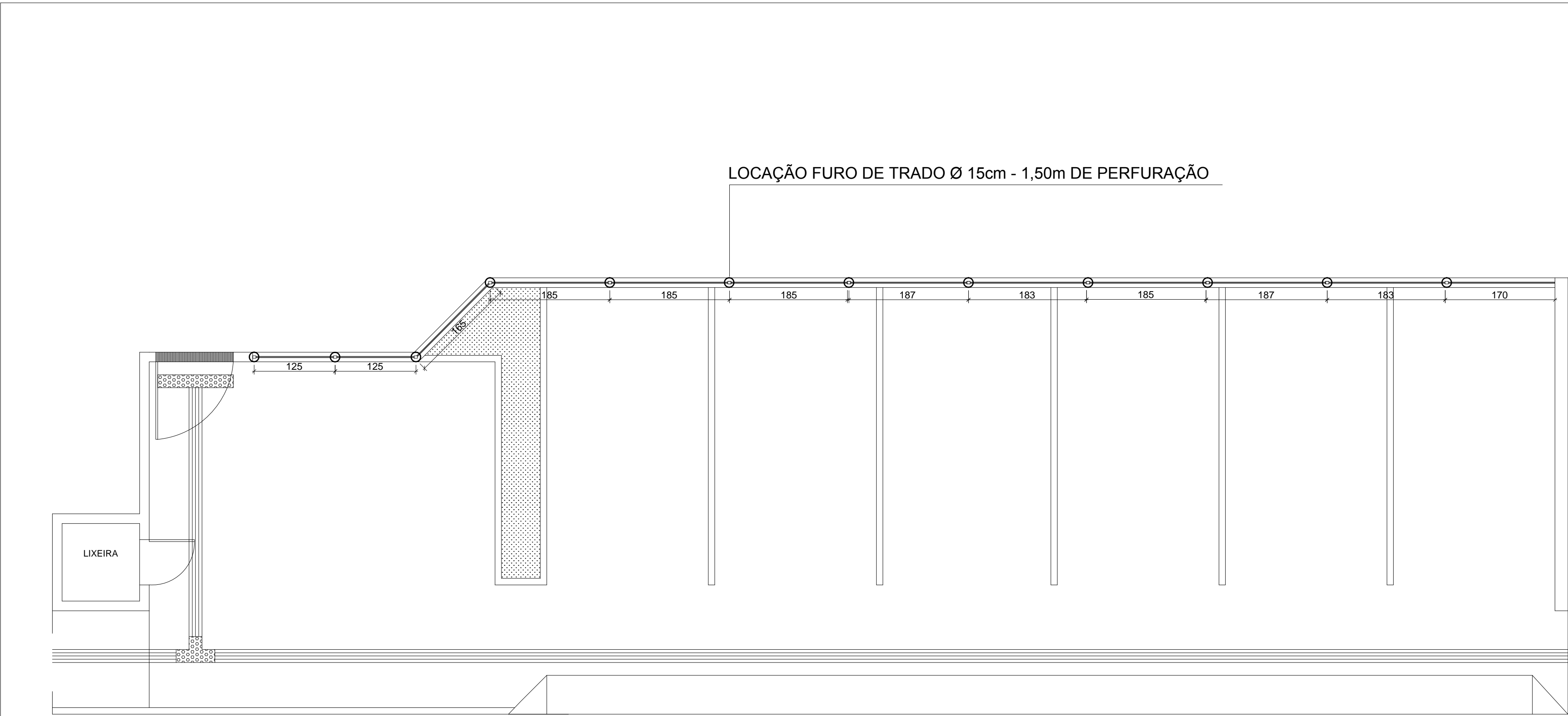
LOCAÇÃO FURO DE TRADO ESCALA 1:50
